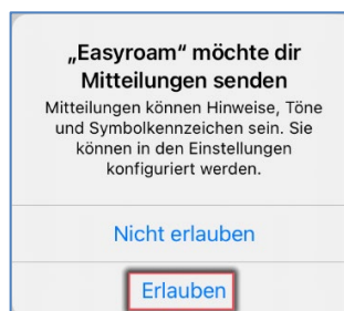
Abbildung 4: Zugriff erlauben
